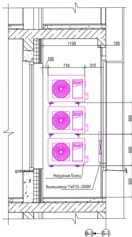
Разрез 2-2
