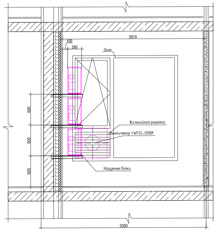
Разрез 1-1
